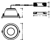
DL CMFT ZB D200 P 30W 93040 U19
