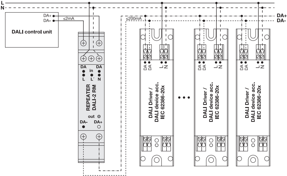
Wiring diagram /Anschluss-Schema 8) DALI mode 9)
