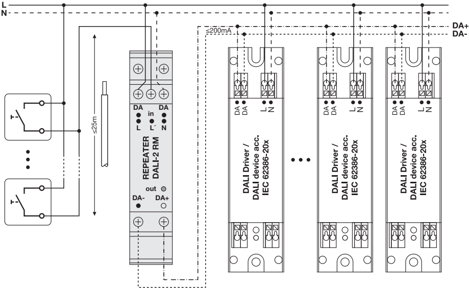
Wiring diagram /Anschluss-Schema 8) Push-DIM mode 10)
