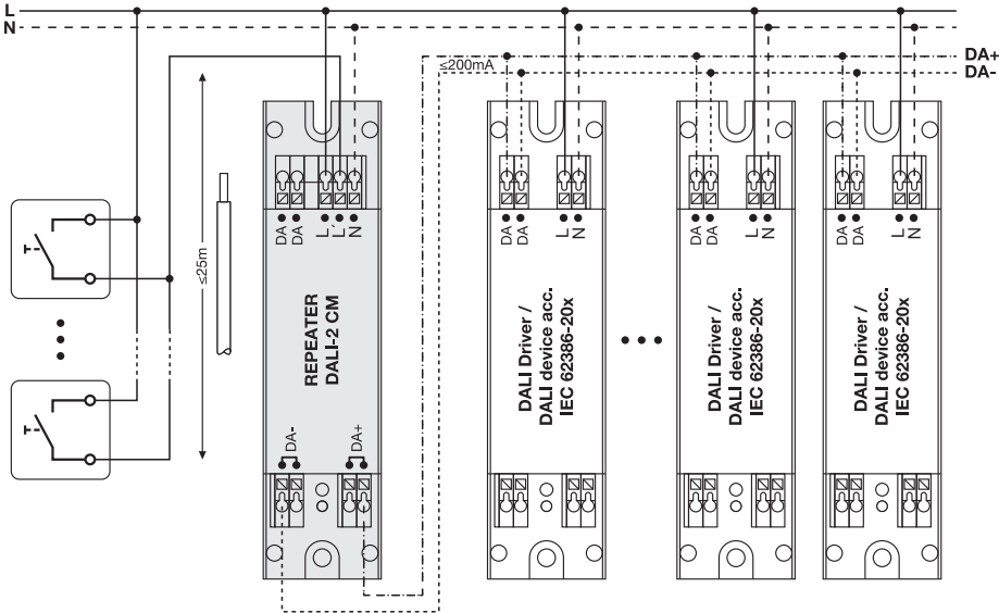
Wiring diagram /Anschluss-Schema 6) Push-DIM mode 8)
