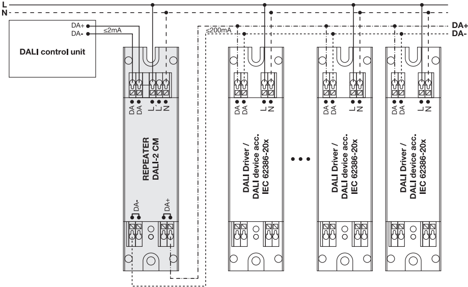
Wiring diagram /Anschluss-Schema 6) DALI mode 7)
